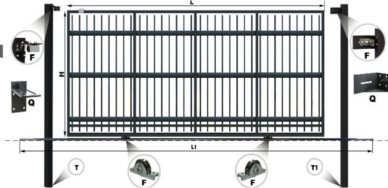
Poartă Glisantă /ZnT/ GP/80x20
