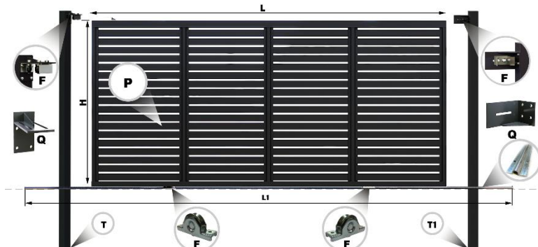
Poartă Glisantă /ZnT/ GP-O/80 1870x4000/20- 6250 lei
